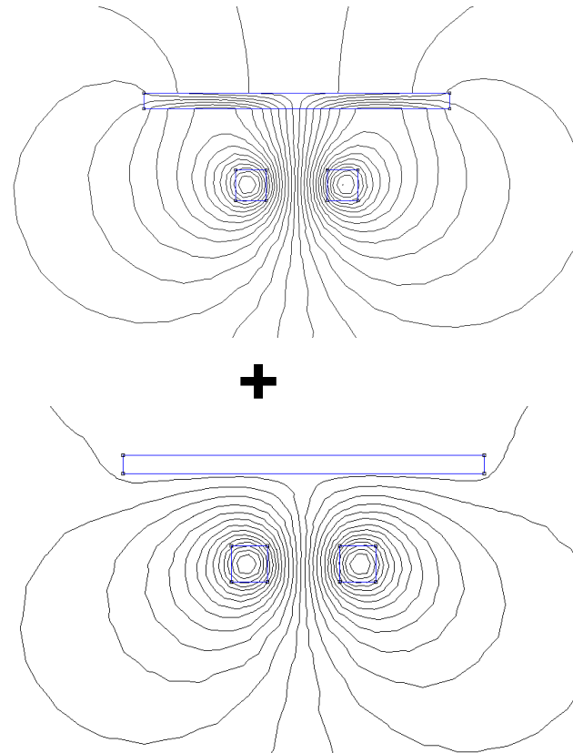
Schermo Ferromagnetico
